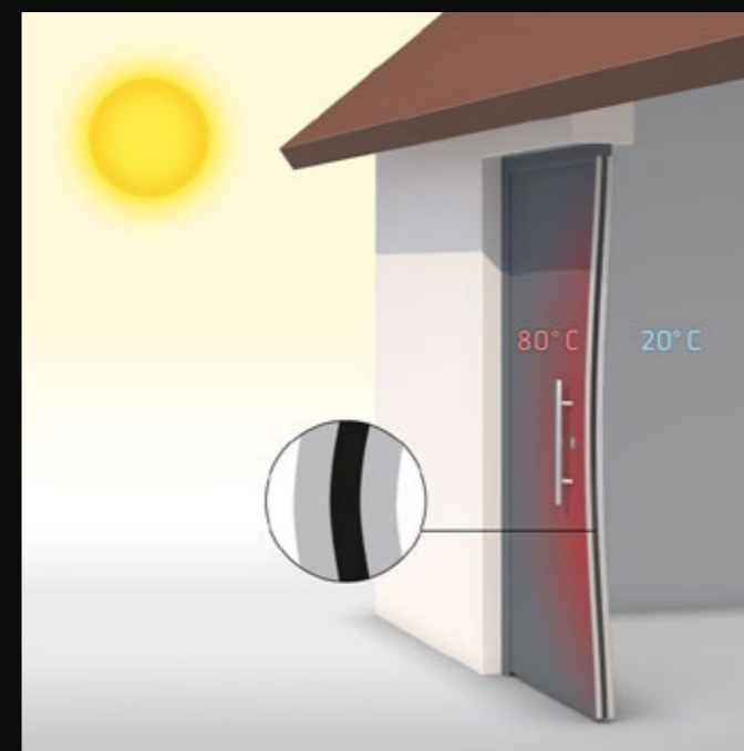
La diferencia de temperatura provoca una deformación en la puerta de aluminio con perfil aislante normal.
