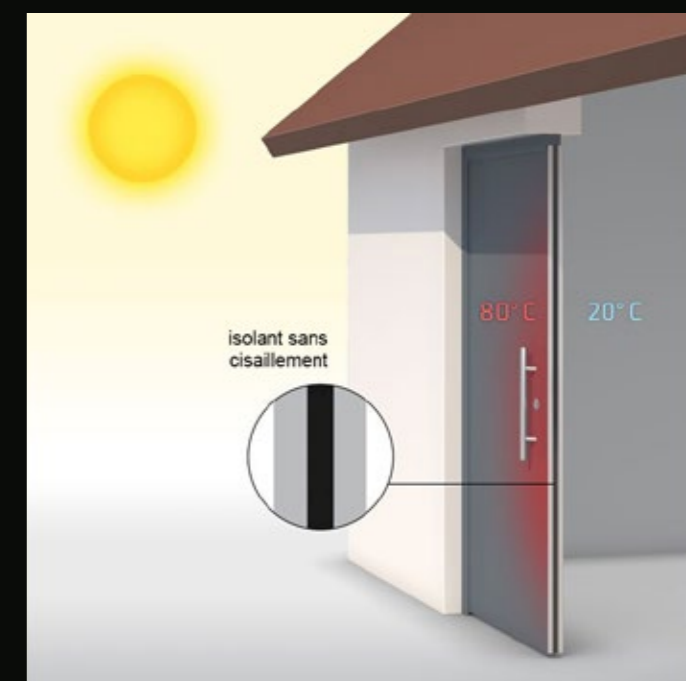
Avec le profilé isolant sans cisaillement, la zone isolante mobile compense les différentes dilatations longitudinales de la face intérieure et extérieure.
