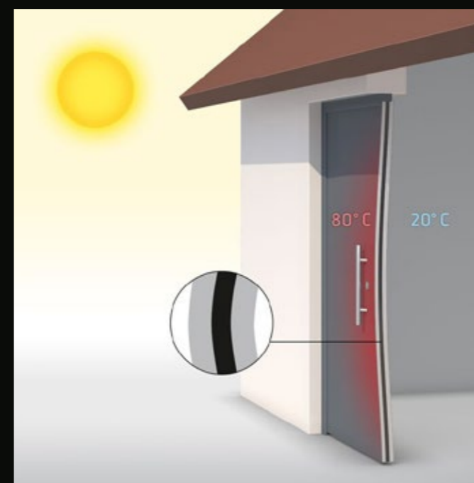
Avec un profilé isolant normal, la différence de température provoque une déformation de la porte en aluminium.
