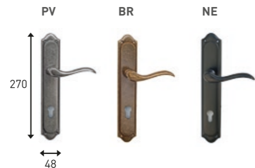
REF. 25 POIGNÉE PVC A92
